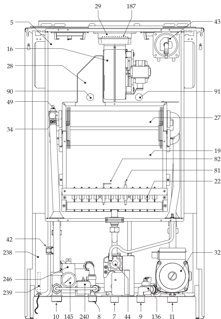
Вид спереди
