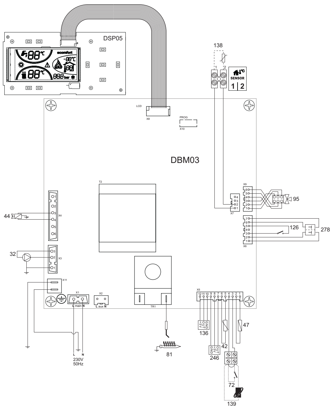
рис. 26 - Электрическая схема
