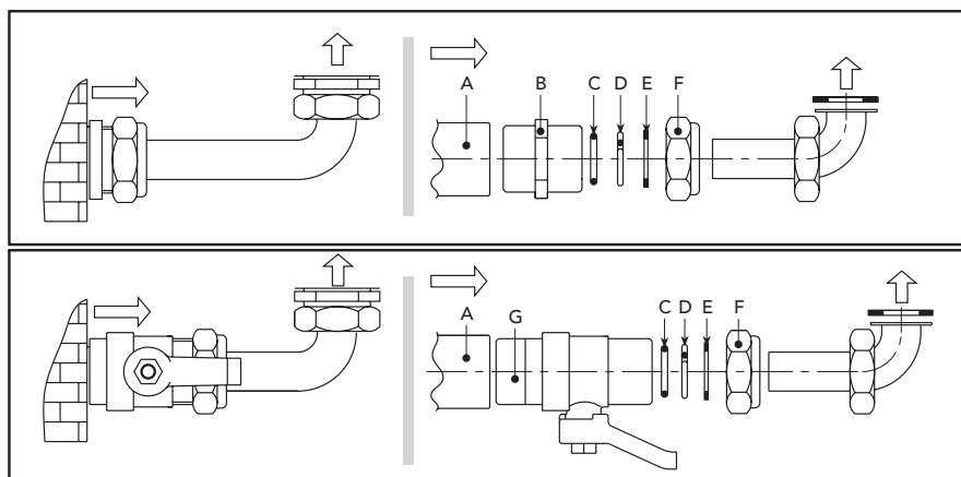
рис. 18 - Соединительный комплект
