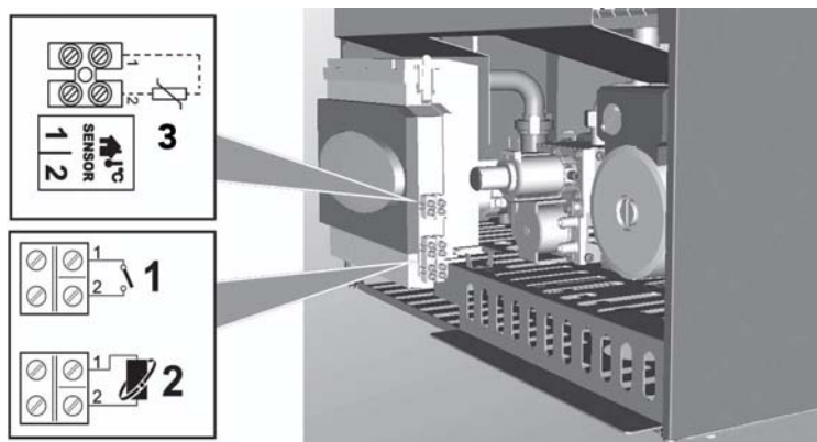
рис. 19 - Доступ к клеммной коробке
