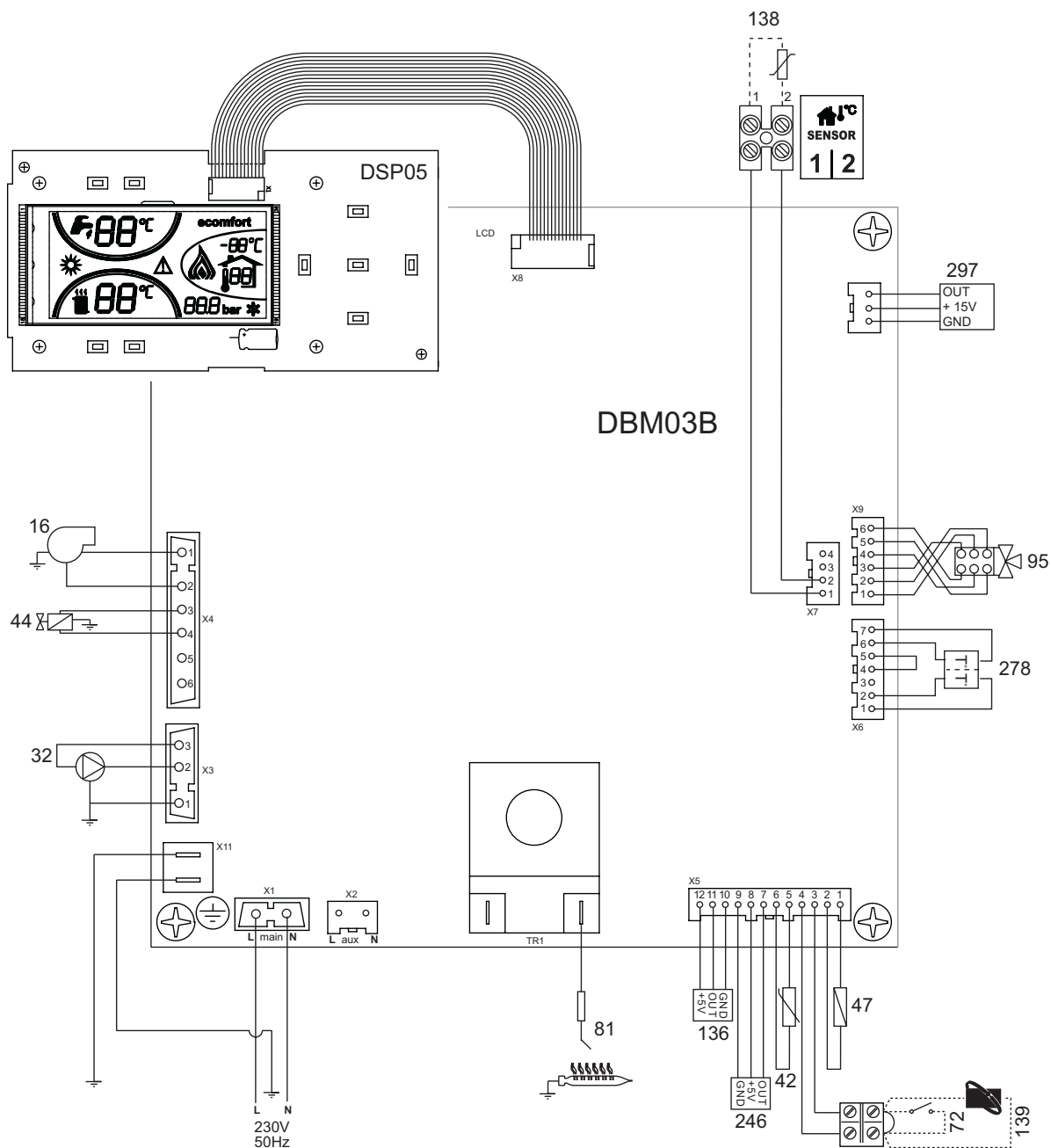
рис. 33 - Электрическая схема
