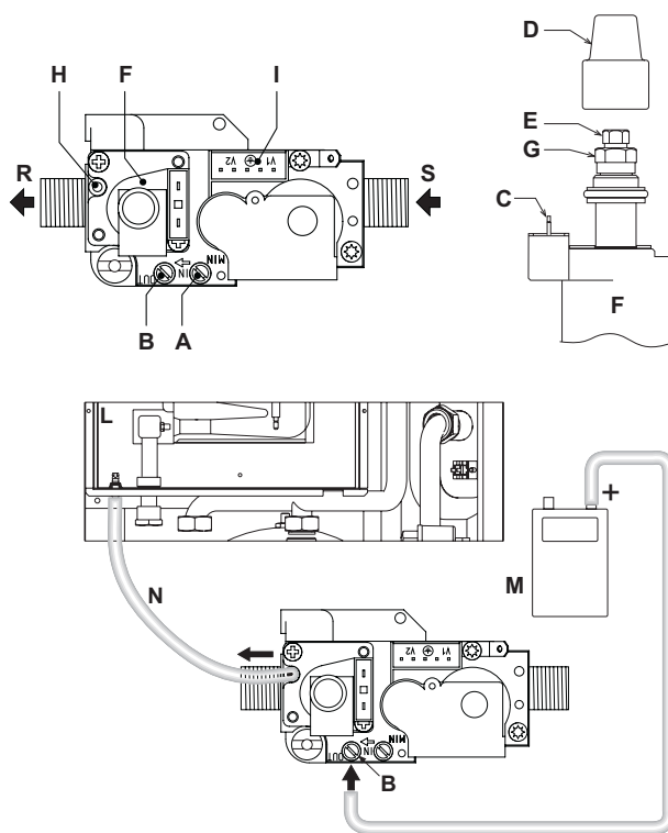
рис. 27 - Газовый клапан
