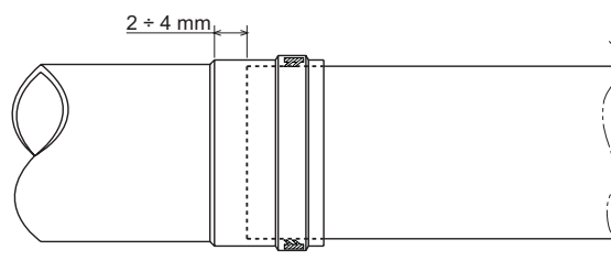
рис. 20 - Тепловое расширение
