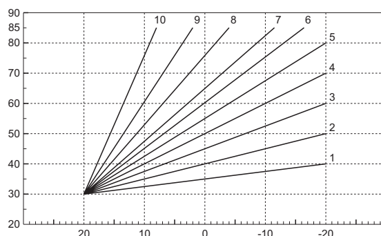
рис. 14 - Компенсационные характеристики
