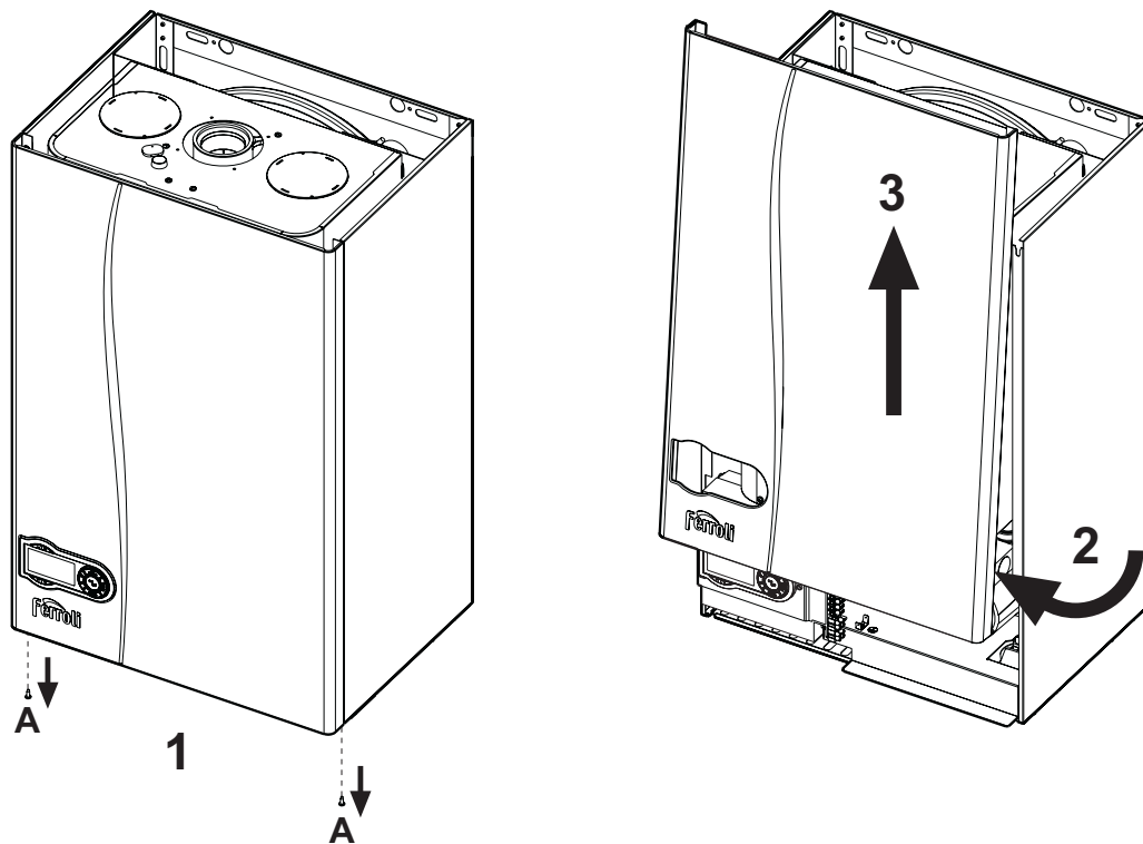
рис. 28 - Снятие кожуха
