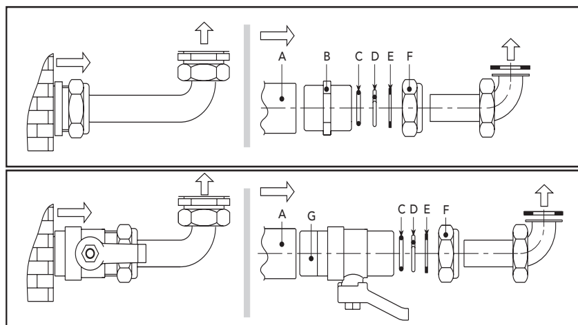
рис. 18 - Соединительный комплект
