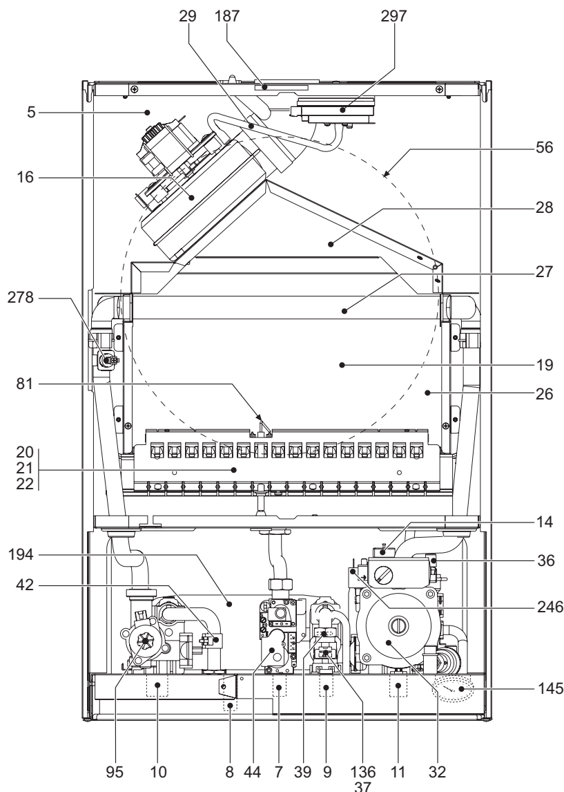
рис. 31 - Общий вид
