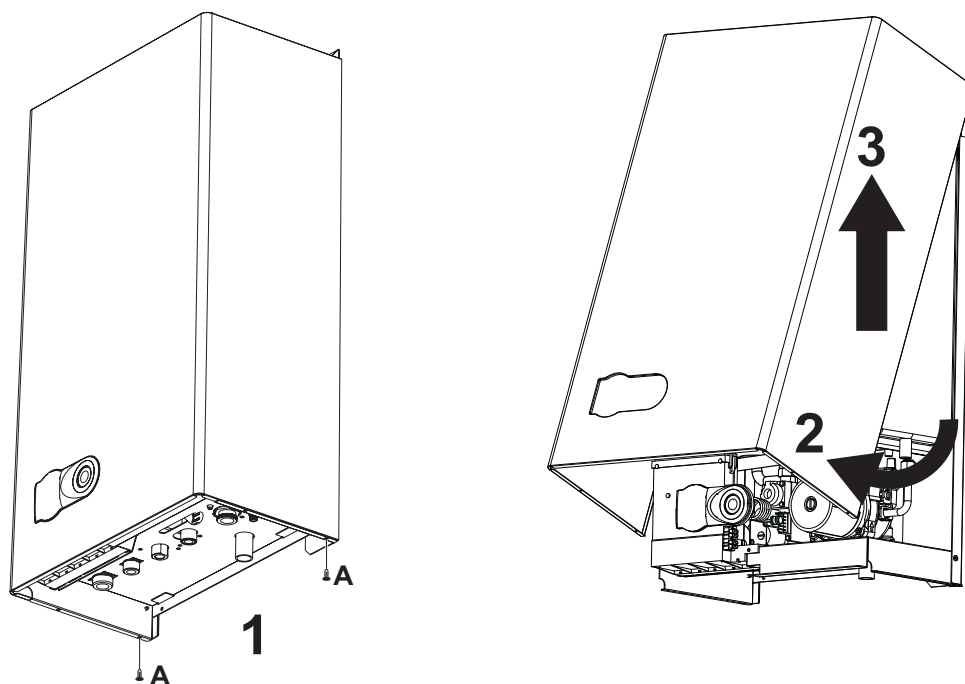
рис. 16 - Снятие кожуха
