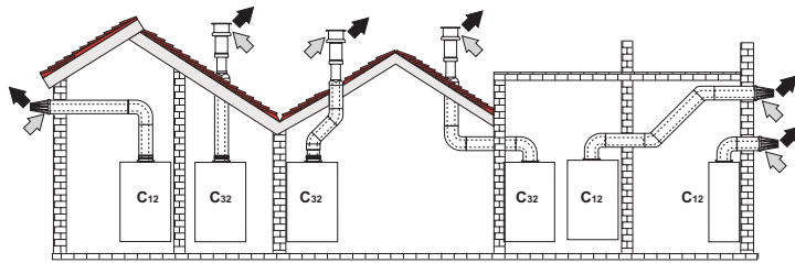
мал. 21 - Приклад підключення за допомогою співісних (коаксialних) труб ( = Повітря / = Відпрацьовані гази)
