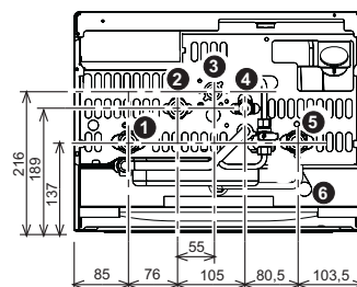
fig. 17 - Attacchi idraulici
