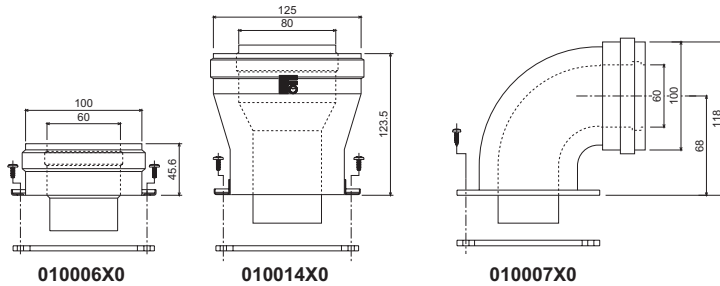
мал. 22 - Початкові елементи для коаксialних трубопроводів
