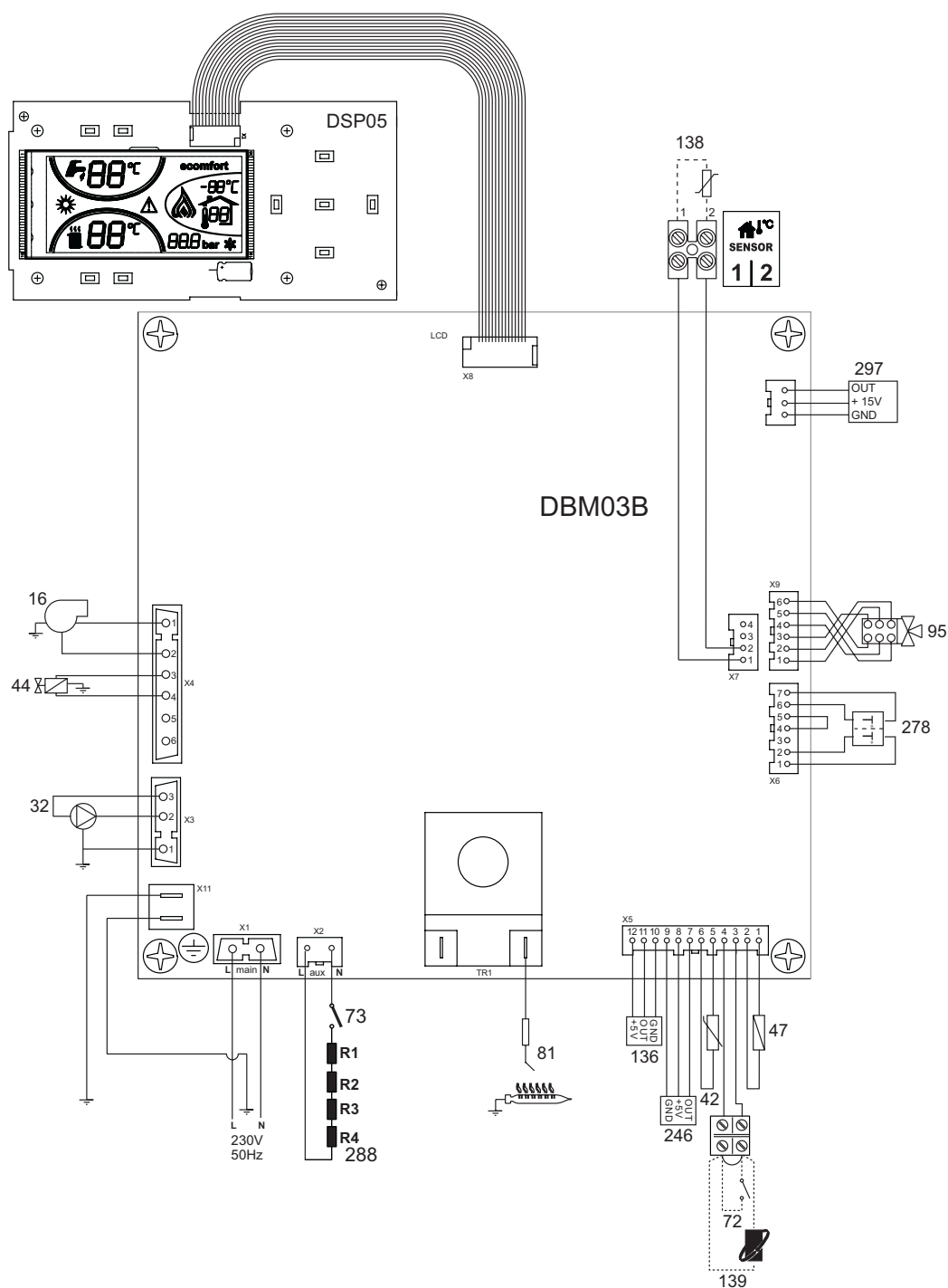
fig. 39 - Schéma électrique
