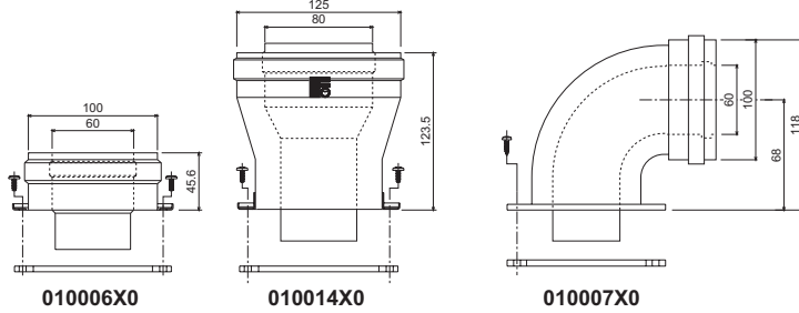
şek. 22 - Koaksiyal kanallar için çıkış aksesuarları
