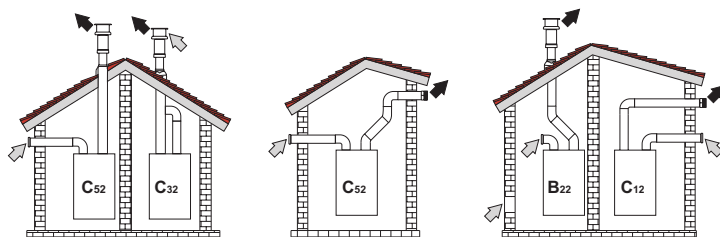
мал. 23 - Приклад підключення за допомогою відокремлених труб ( = Повітря / = Відпрацьовані гази)
