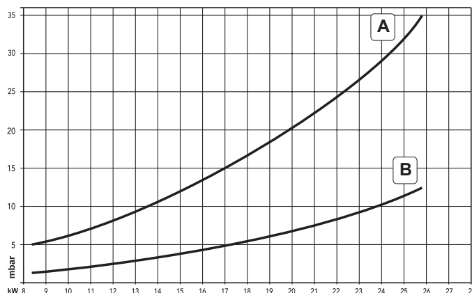
fig. 33 - Diagramma pressione/potenza DIVAtop MICRO F 24
