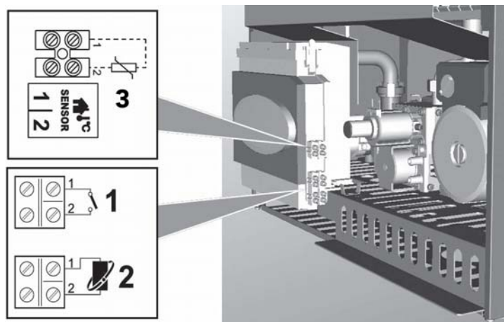
fig. 20 - Acceso a la regleta de conexiones
