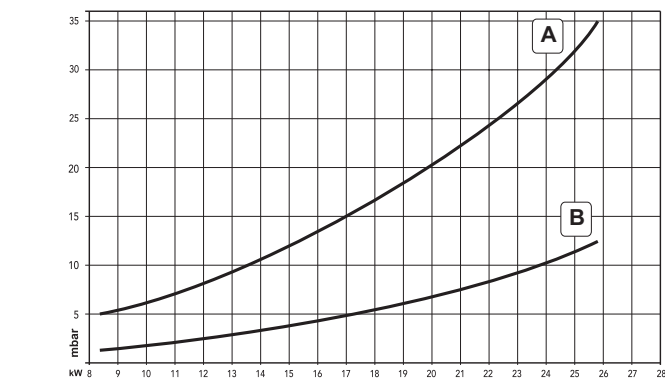
рис. 33 - Диаграммы давление - мощность DIVAtop MICRO F 24
