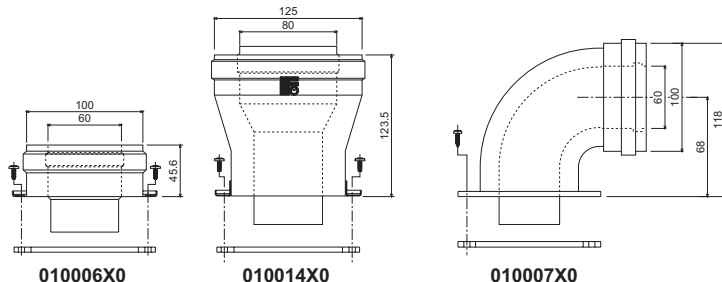
fig. 22 - Accesorii de plecare pentru conducte coaxiale
