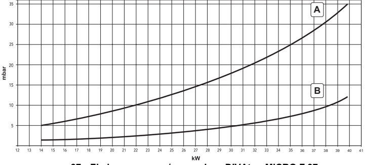
мал. 37 - Діафрагма тиску/потужність DIVAtop MICRO F 37
