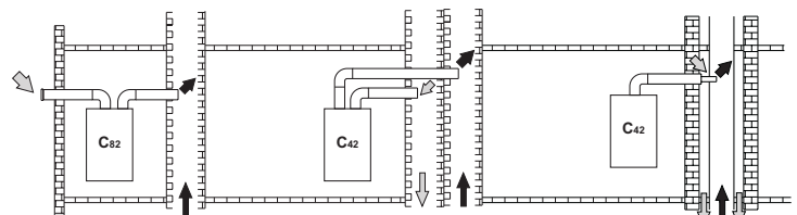
мал. 25 - Приклад підключення до димарів ( = Повітря / = Відпрацьовані гази)
