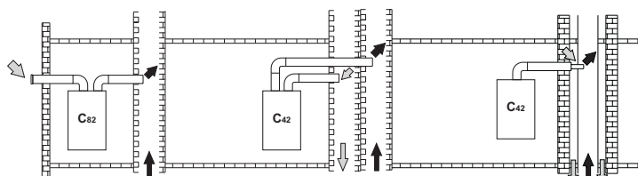
fig. 25 - Ejemplos de conexión a chimeneas (→ = aire / → = humos)
