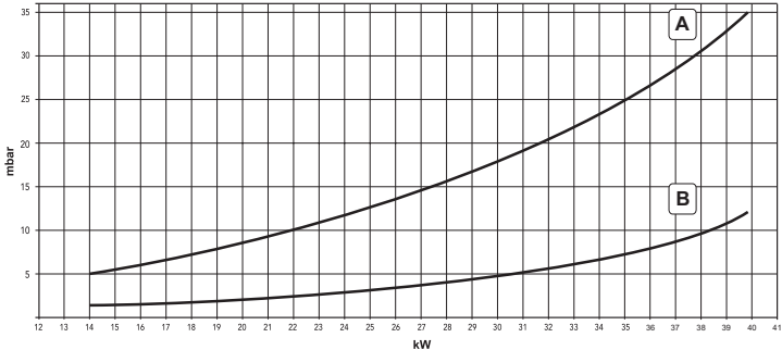
fig. 37 - Diagrama presión / potencia DIVAtop MICRO F 37
