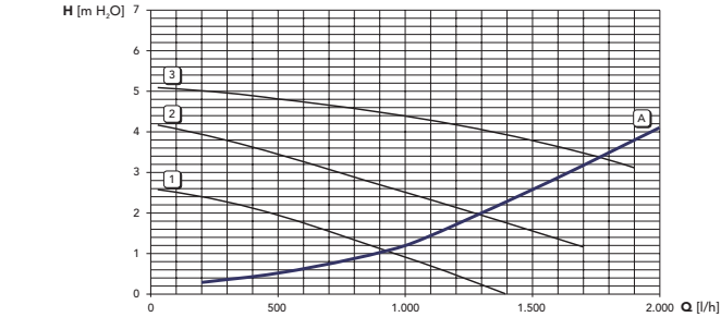
fig. 34 - Pertes de charge / pression circulateurs DIVAtop MICRO F 24
