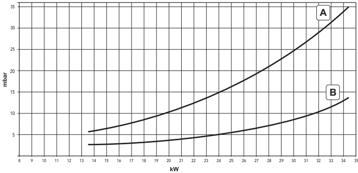
fig. 35 - Diagrammes pression - puissance DIVAtop MICRO F 32
