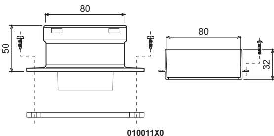
мал. 24 - Початковий елемент для відокремлених трубопроводів
