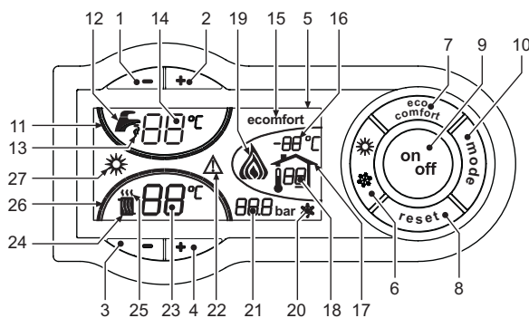
рис. 1 - Панель управления
