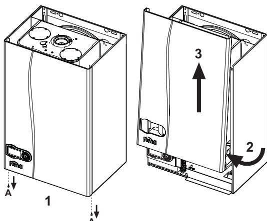
fig. 28 - Deschiderea carcasei
