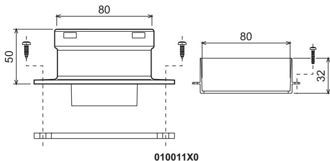
fig. 24 - Accesorii de plecare pentru conducte separate
