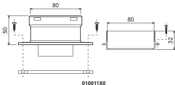
fig. 24 - Accesorio inicial para conductos separados
