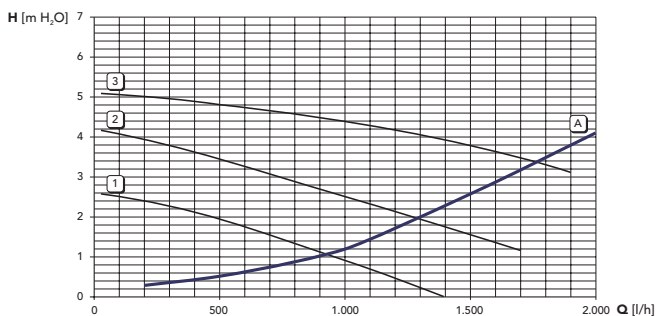
fig. 34 - Pierderi de sarcină / înălțime de pompare pompe de circulație DIVAtop MICRO F 24
