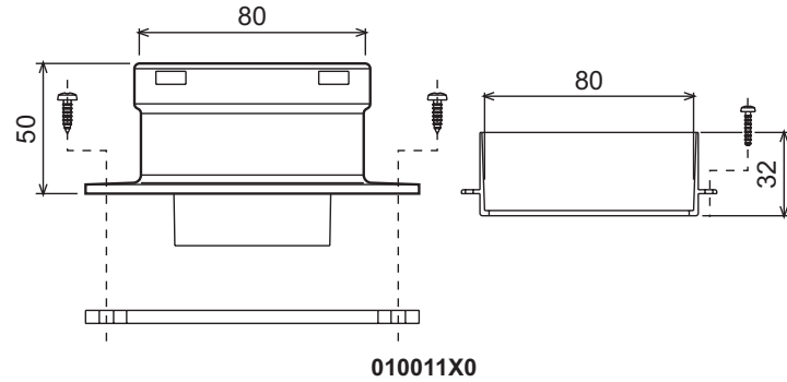
şek. 24 - Ayrı kanallar için çıkış aksesuarları
