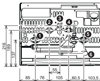
fig. 17 - Conexiones hidráulicas
