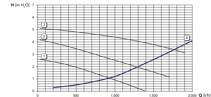
рис. 34 - Потери напора циркуляционных насосов DIVAtop MICRO F 24
