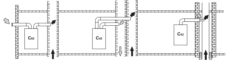
şek. 25 - Duman kanalına bağlantı örneği (⇨ = Hava / ⇨ = Duman)
