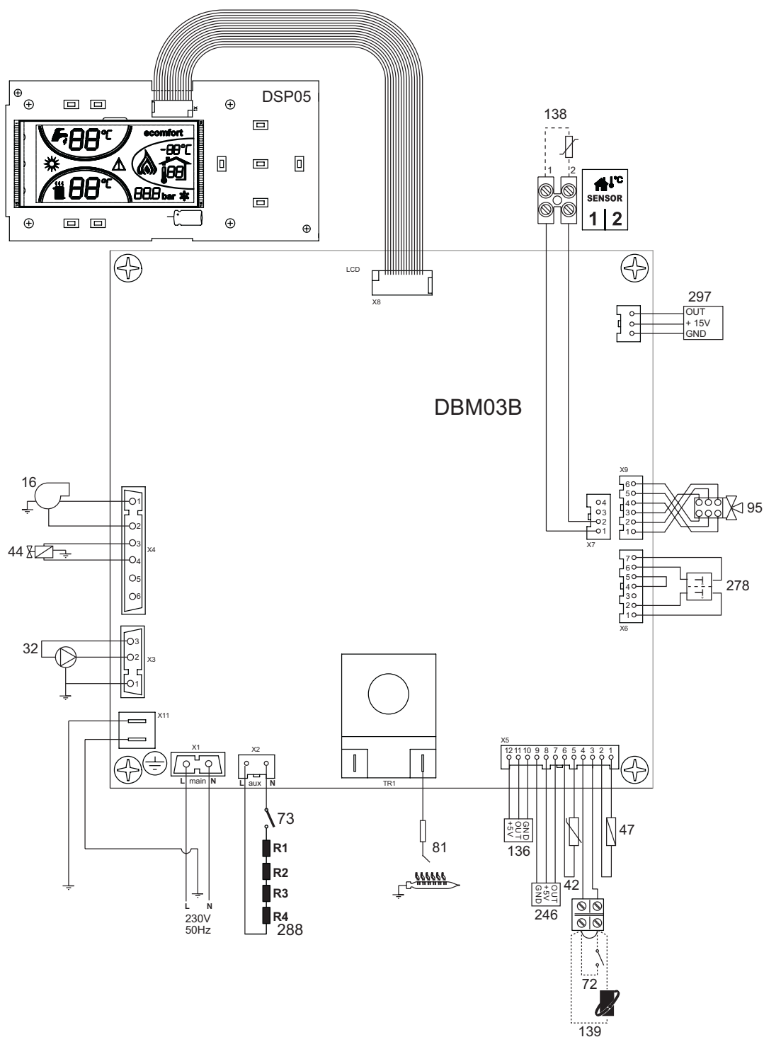
fig. 39 - Esquema eléctrico
