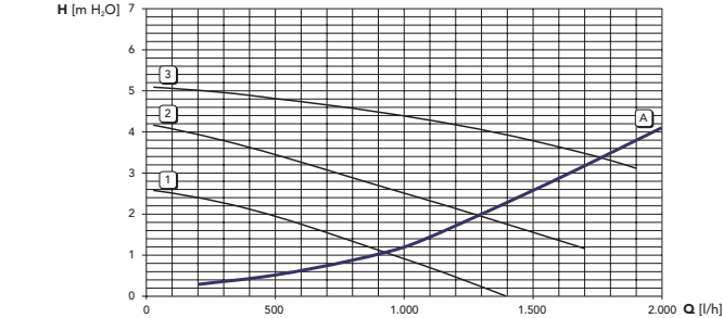
fig. 34 - Pérdidas de carga / carga hidrostática de las bombas de circulación DIVAtop MICRO F 24
