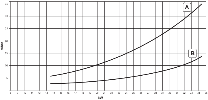
мал. 35 - Діафрагма тиску/потужність DIVAtop MICRO F 32
