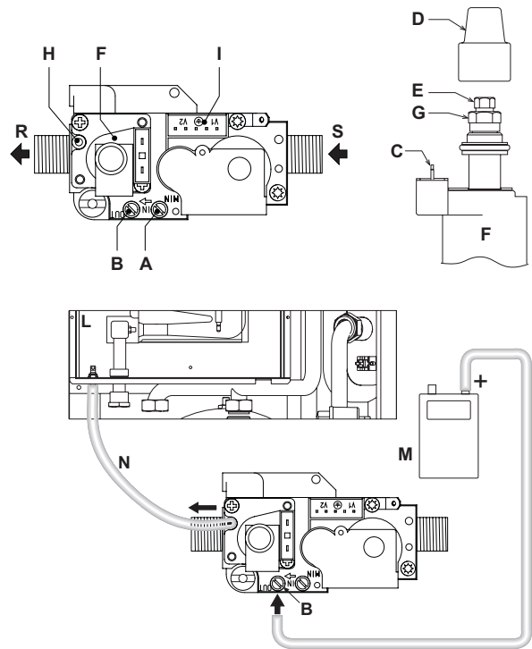
рис. 27 - Газовый клапан
