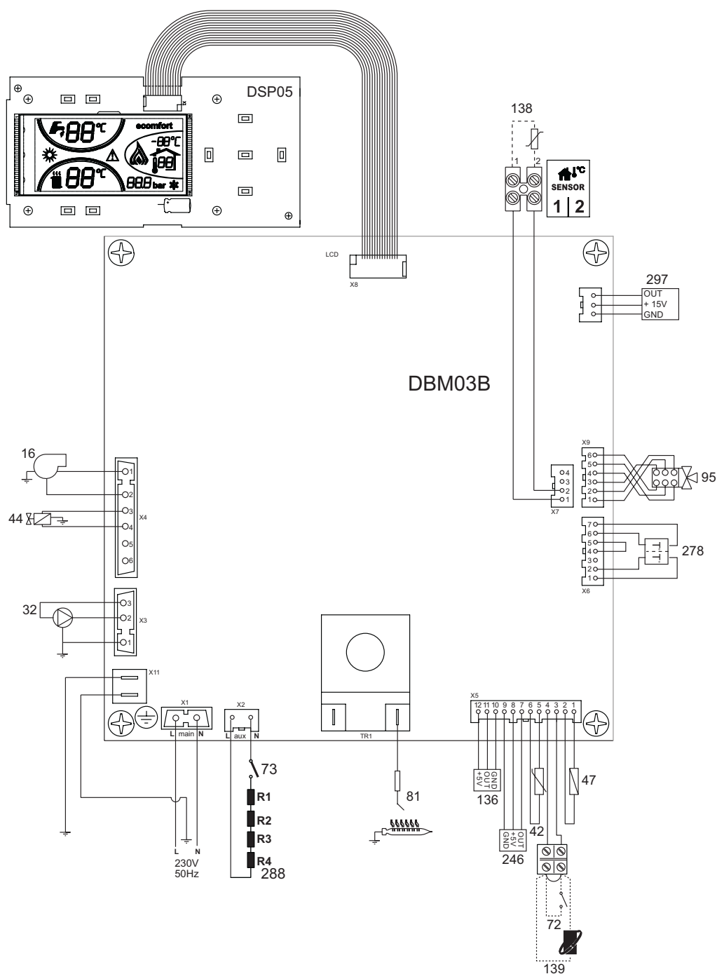
fig. 39 - Schemă electrică
