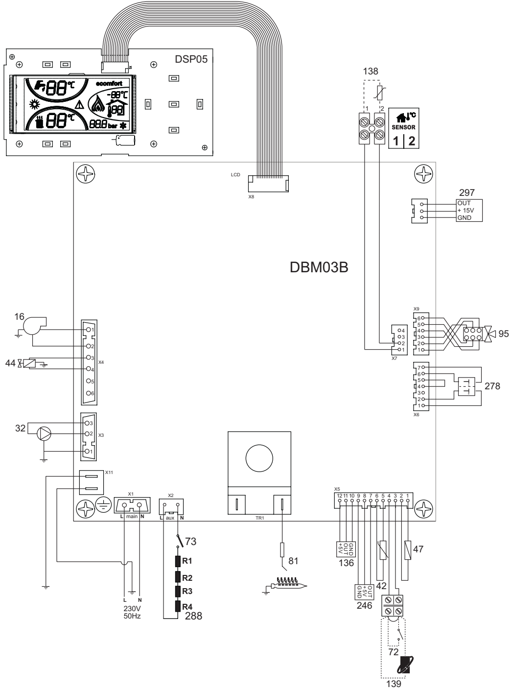
şek. 39 - Elektrik şeması
