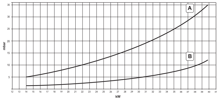
fig. 37 - Diagramă presiune/putere DIVAtop MICRO F 37
