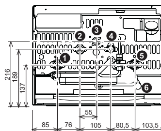
fig. 17 - Racordurile hidraulice
