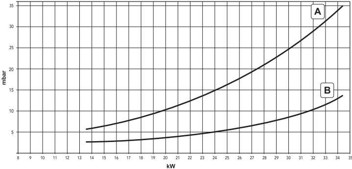
fig. 35 - Diagrama presión / potencia DIVAtop MICRO F 32
