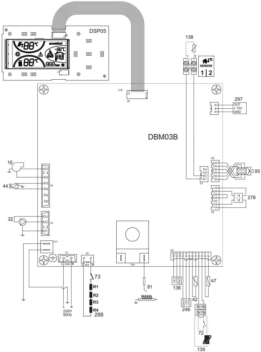
fig. 39 - Wiring diagram
