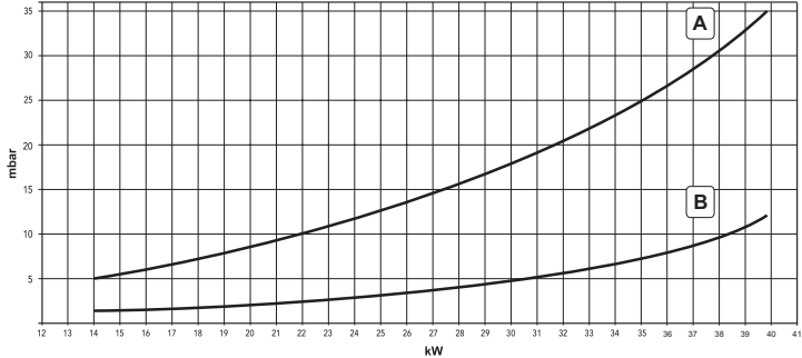
fig. 37 - Diagrammes pression/puissance DIVAtop MICRO F 37
