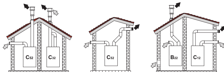
fig. 23 - Exemples de raccordements avec conduits séparés (⇄ = Air / ⇄ = Fumées)
