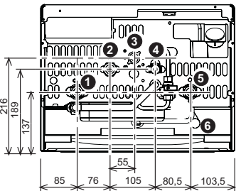
рис. 17 - Гидравлические соединения
