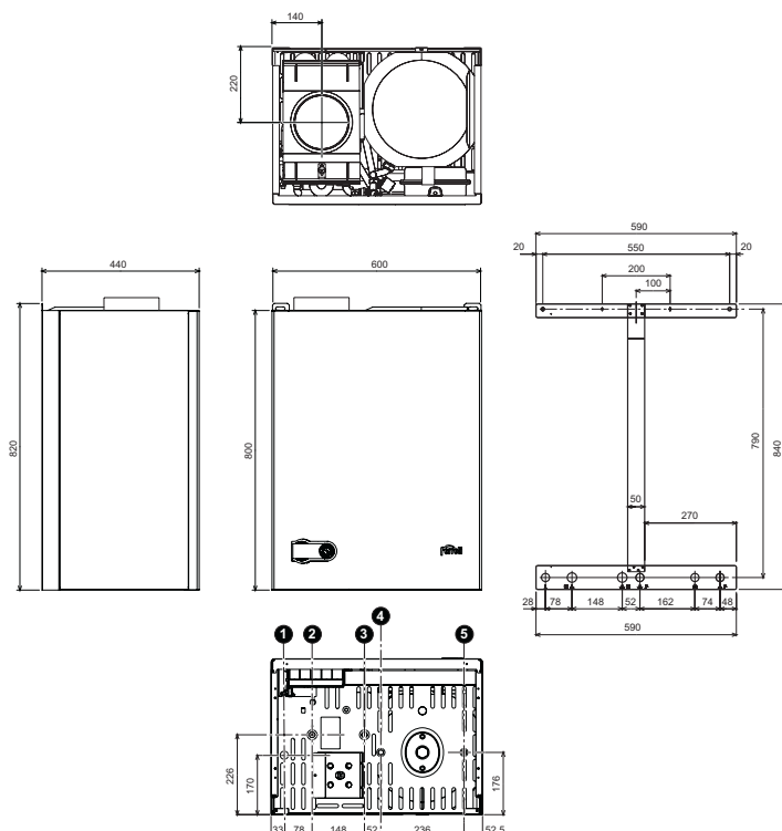
рис. 22 - Габаритные размеры и присоединения
