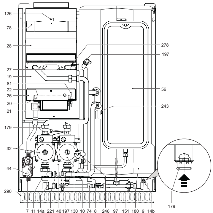
рис. 23 - Общий вид
