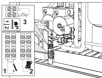
рис. 18 - Доступ к блоку зажимов
