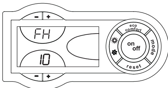
рис. 5 - Включение котла
