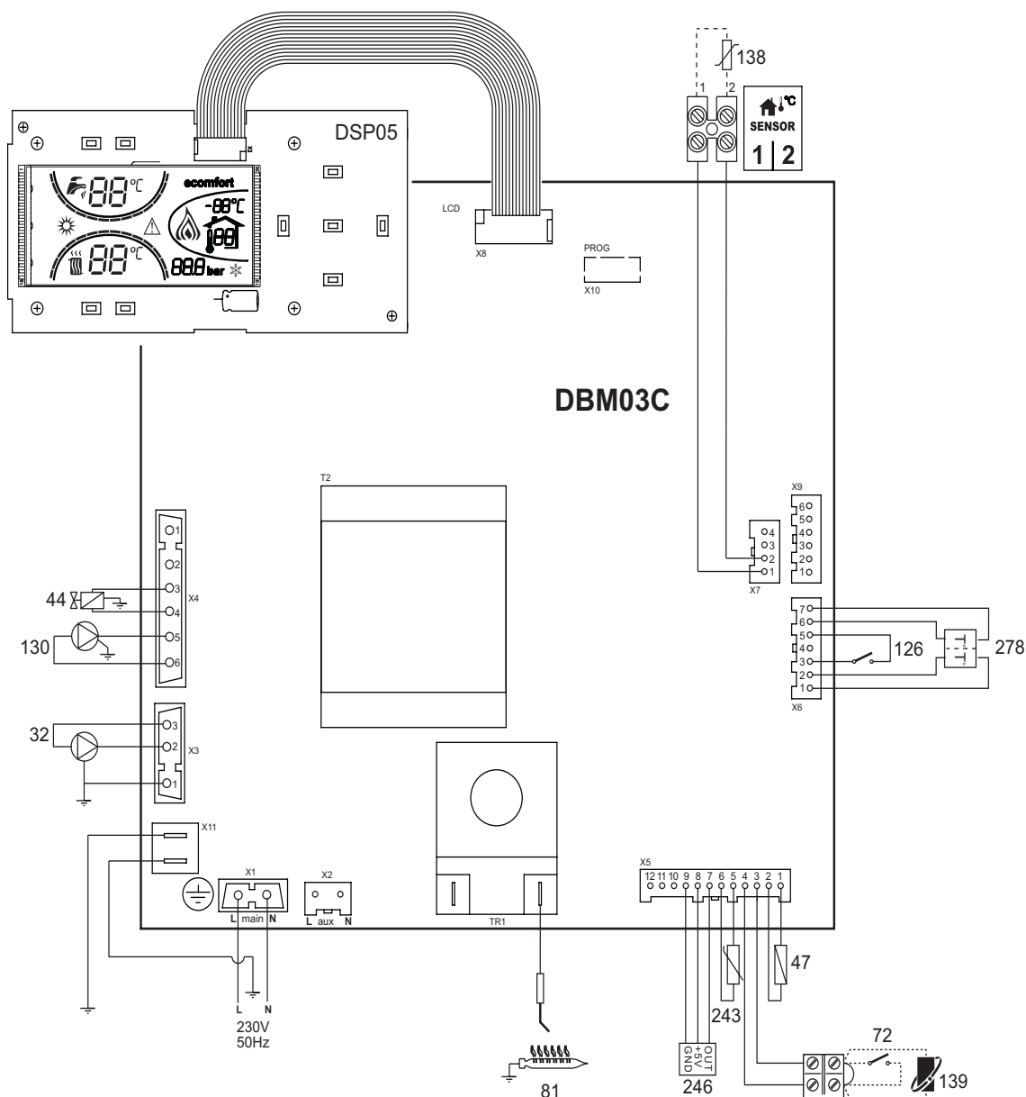
рис. 25 - Электрическая схема
