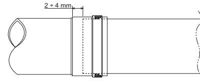
рис. 19 - Тепловое расширение
