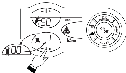
рис. 26 - Режим TEST (мощность отопления = 100%)
