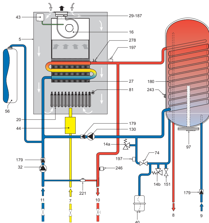
рис. 32 - Схема системы отопления и ГВС
