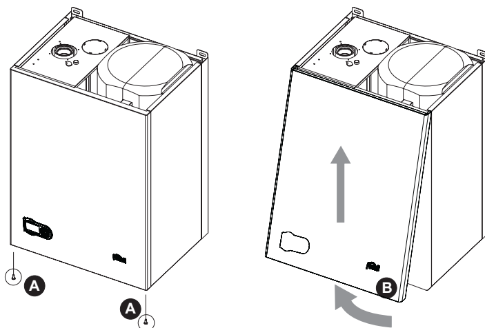
рис. 28 - Демонтаж кожуха
