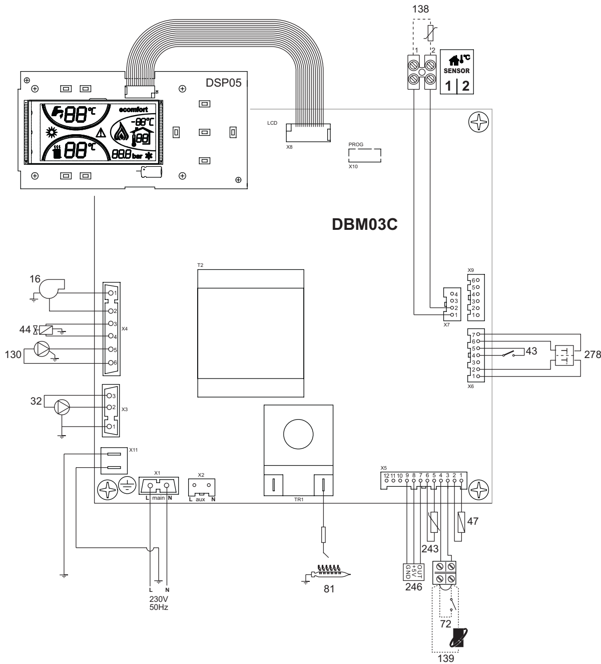
рис. 37 - Электрическая схема
