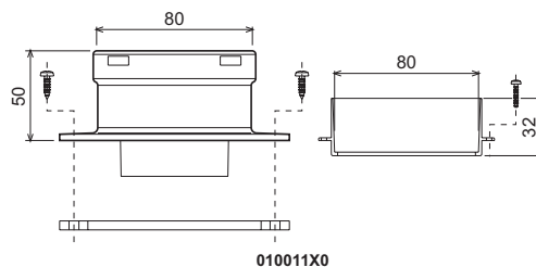
рис. 24 - Соединительный элемент для раздельных труб
