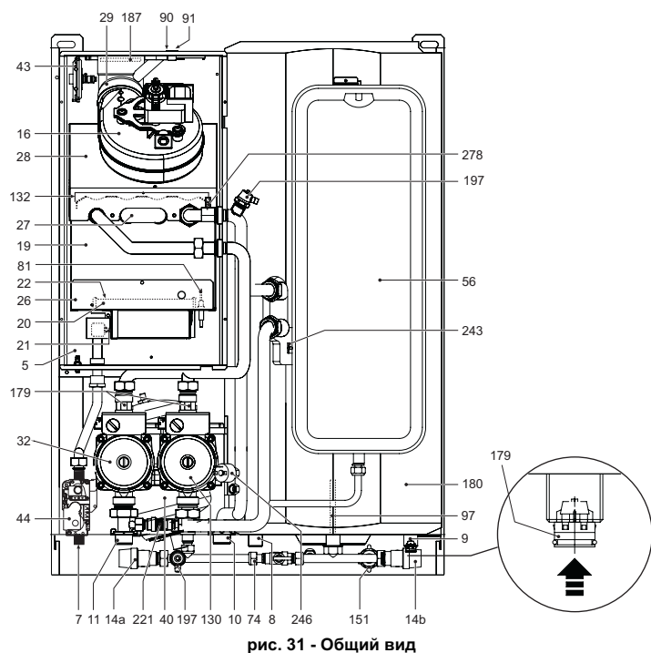
рис. 31 - Общий вид
