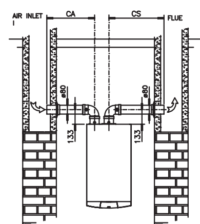
Дымоудаление и воздухозабор из общих каналов
