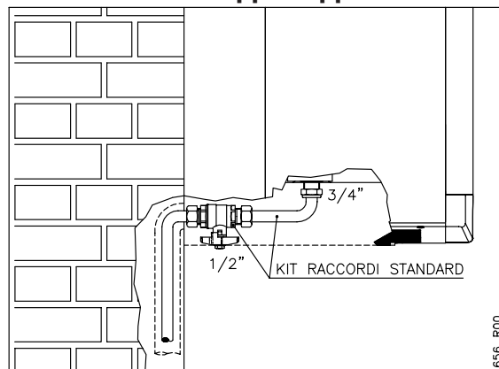
ПРИМЕР ПОДСОЕДИНЕНИЯ
