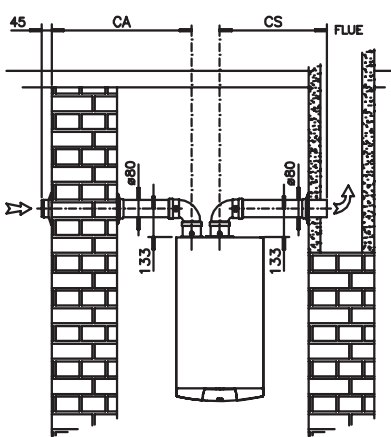
воздухозабор через стену дымоудаление через общий канал
