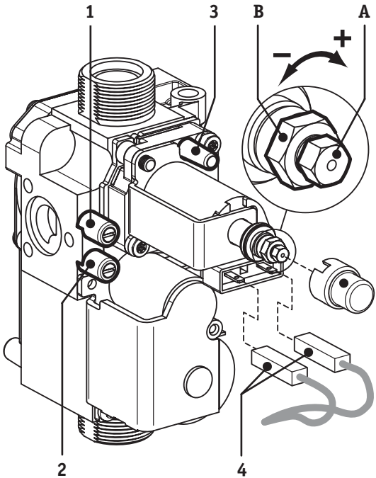
1 Выход газа 2 Вход газа 3 «Vent» (мод. SE) 4 Провода
