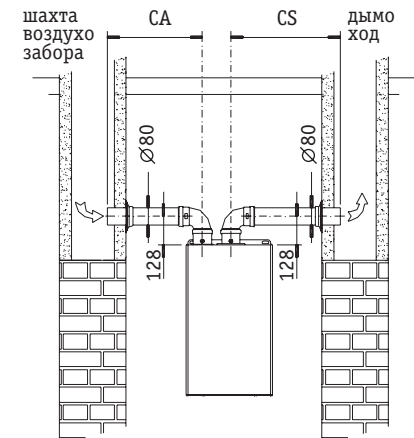
Воздухозабор из вентиляционной шахты, дымоотвод в дымоход
