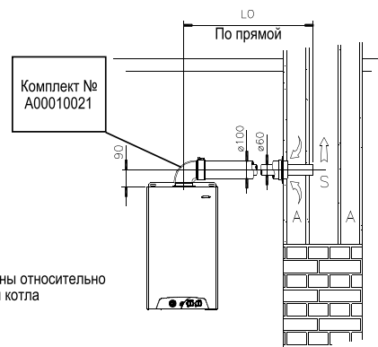
ГОРИЗОНТАЛЬНОЕ КОАКСИАЛЬНОЕ ПОДСОЕДИНЕНИЕ К КОЛЛЕКТИВНОЙ КОАКСИАЛЬНОЙ ШАХТЕ ДЫМОУДАЛЕНИЯ И ВОЗДУХОЗАБОРА SCHIEDEL QUADRO (LAS-СИСТЕМА)
