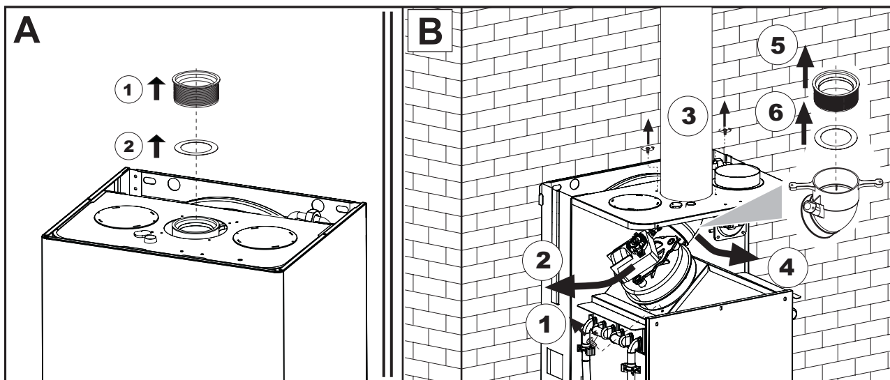
рис. 8 - Замена диафрагмы (A = если котел не установлен / B = Если котел и воздухопроводы уже смонтированы)
