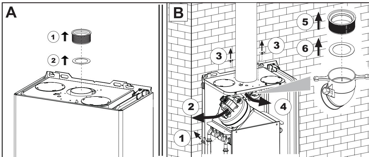
рис. 8 - Замена диафрагмы (А = если котел не установлен / В = Если котел и воздуховоды уже смонтированы)
