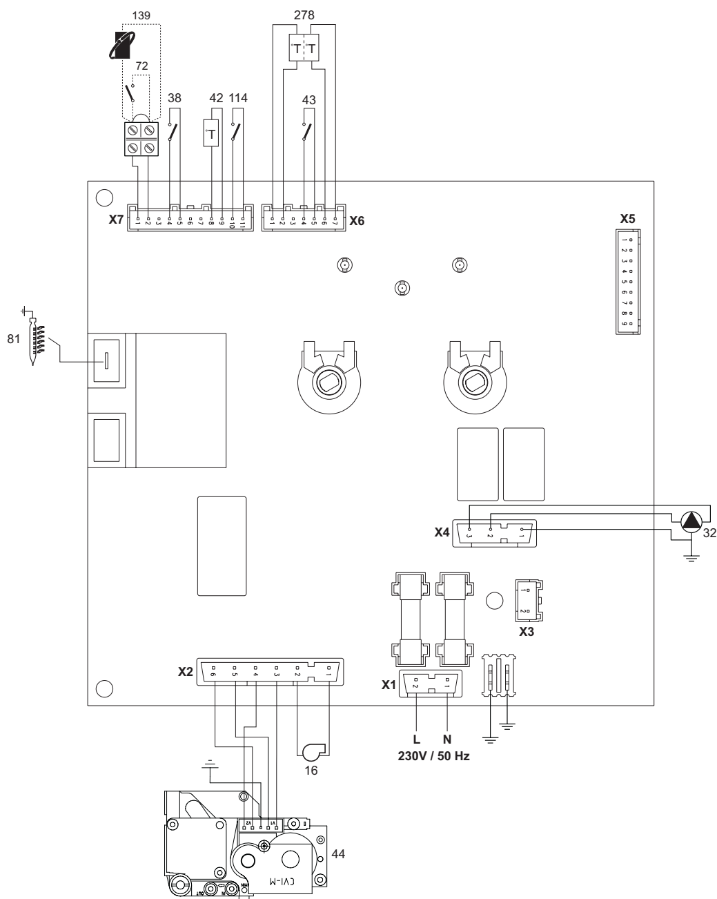
рис. 21 - Электрическая схема
