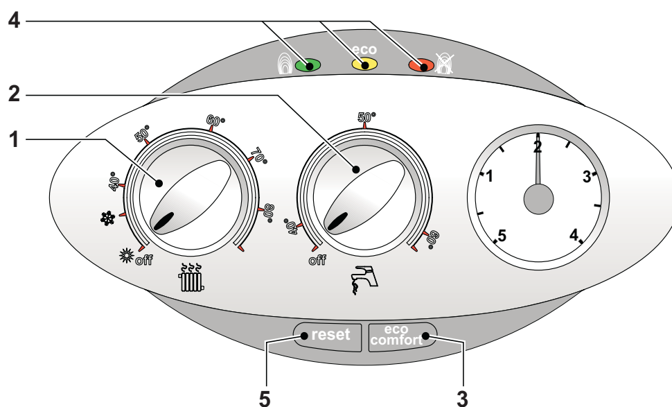
рис. 1 - Панель управления
