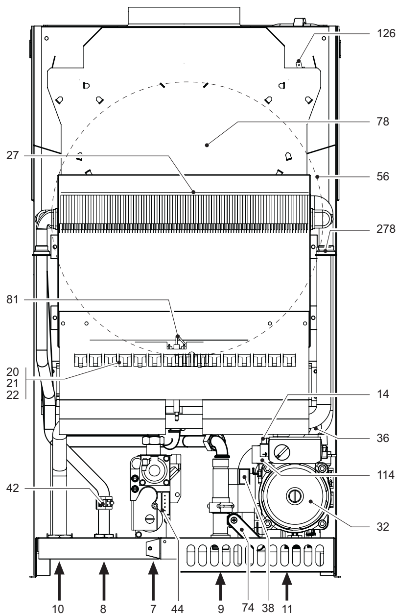
рис. 11 - Общий вид
