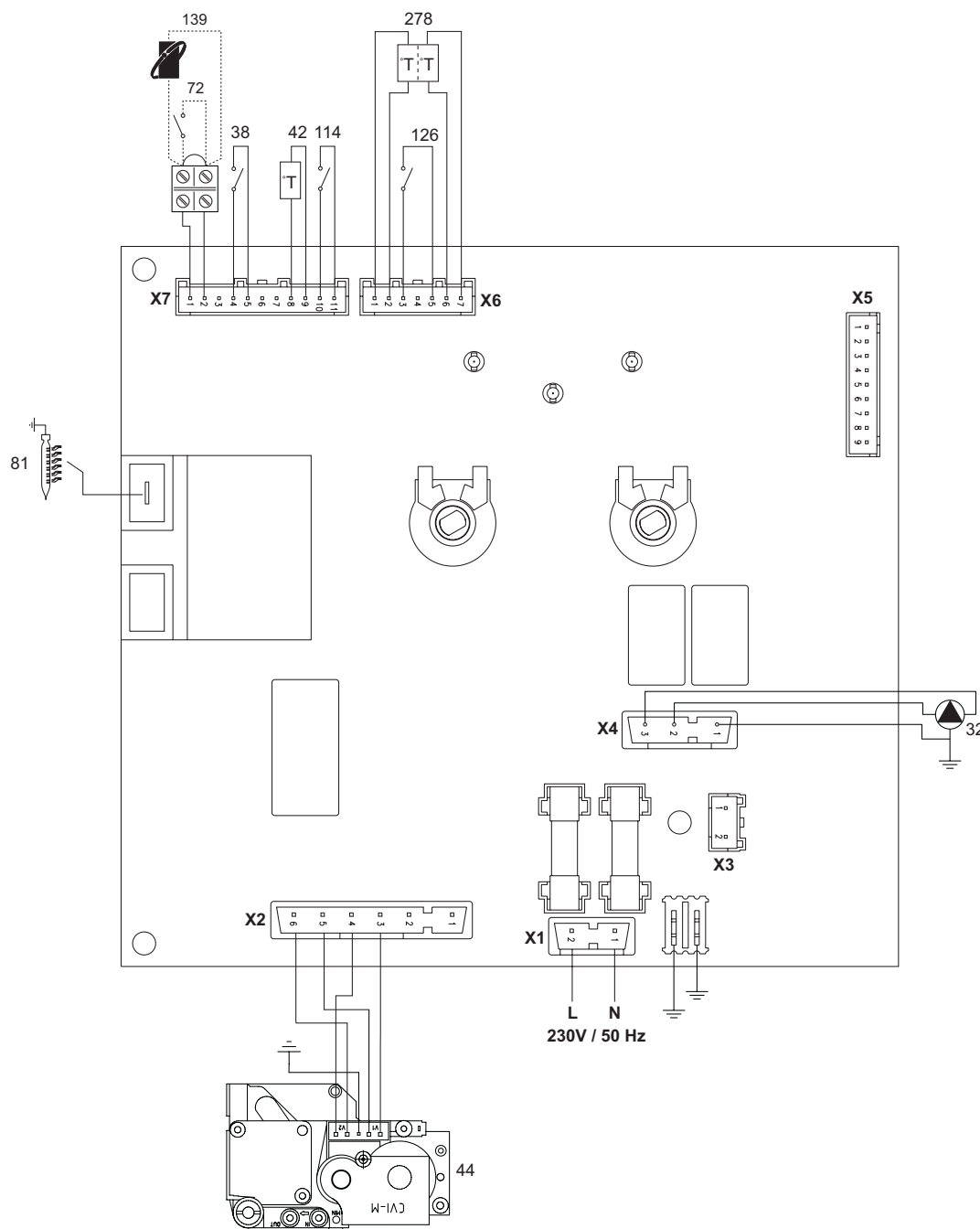
рис. 13 - Электрическая схема
