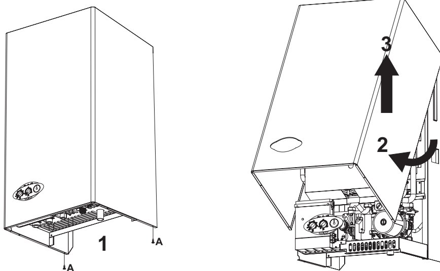
рис. 9 - Демонтаж кожуха
