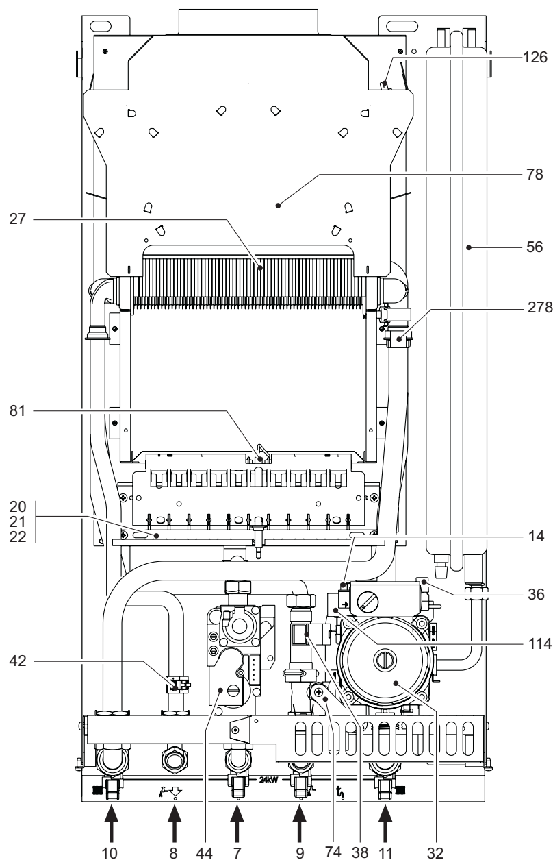
рис. 11 - Общий вид
