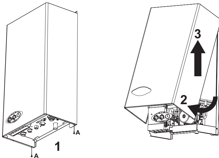
рис. 9 - Снятие кожуха
