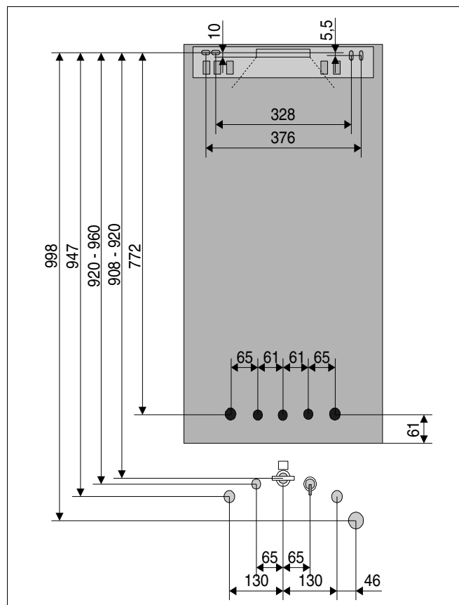
Рис. 11 Совместимость с устройствами Junkers ZWR (комбинированное устройство)
