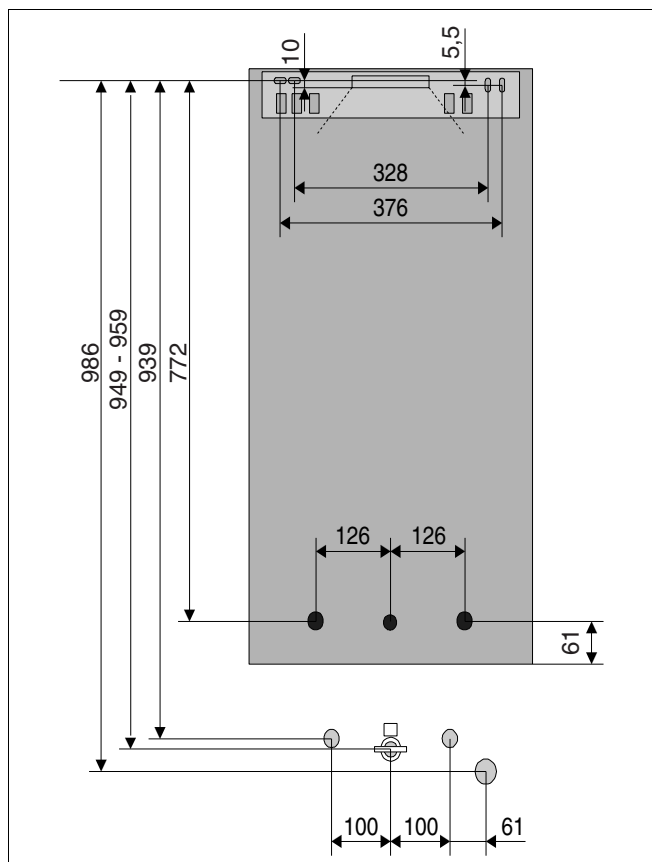
Рис. 10 Совместимость с устройствами Vaillant VC (отдельное устройство)
