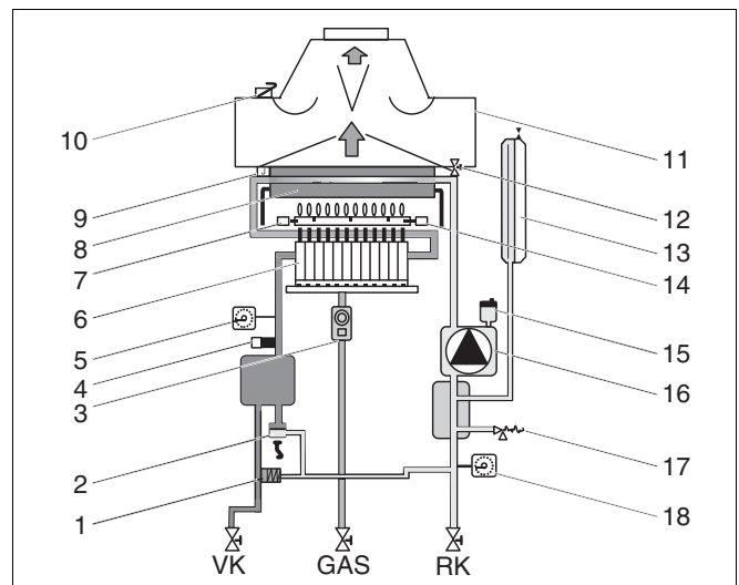
Рис. 2 Конструктивная схема Logamax U104
