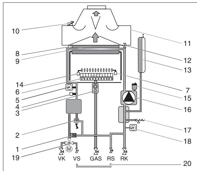
Рис. 4 Конструктивная схема Logamax U004 с 3-ходовым клапаном
