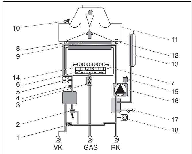
Рис. 1 Конструктивная схема Logamax U004
