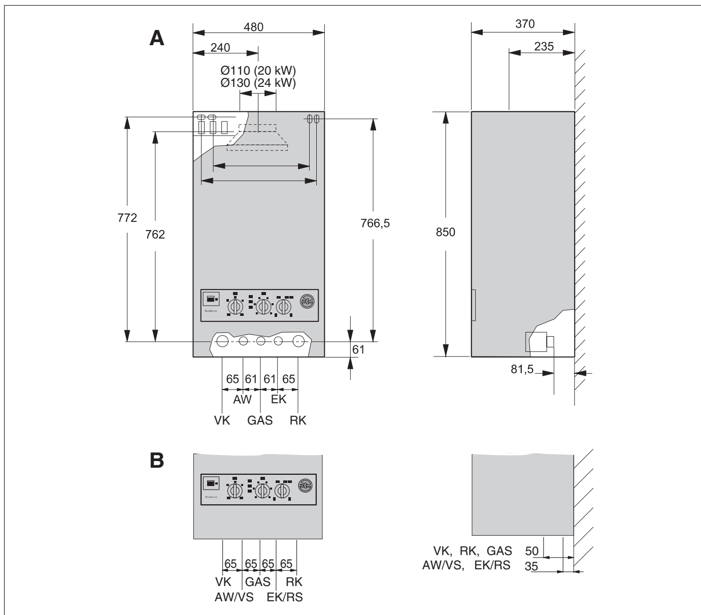
Рис. 8 Габариты настенного водонагревателя
