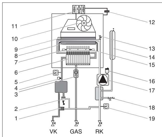
Рис. 2 Конструктивная схема Logamax U102
