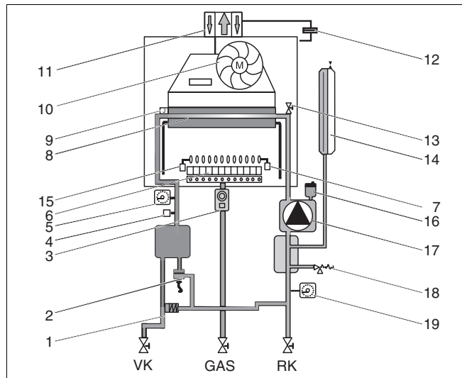
Рис. 1 Конструктивная схема Logamax U002
