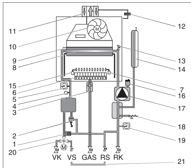
Рис. 4 Конструктивная схема Logamax U002 с 3-ходовым клапаном
