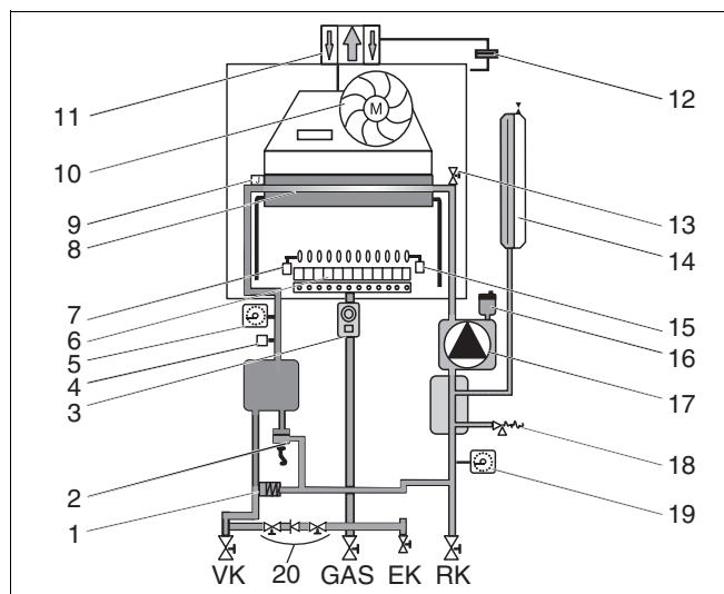
Рис. 3 Конструктивная схема Logamax U002 с разъединителем
