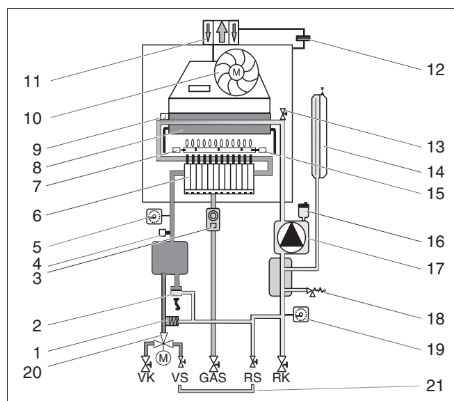
Рис. 5 Конструктивная схема Logamax U102 с 3-ходовым клапаном
