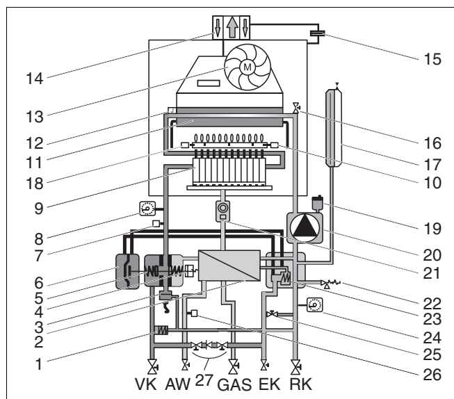
Рис. 7 Конструктивная схема Logamax U102K с разъединителем (FR) или устройством наполнения (IT/TR)
