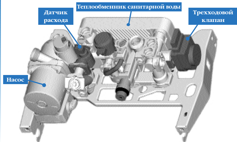
Гидравлический блок
