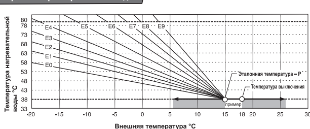
Кривые характеристики погоды
