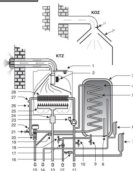
Рабочая схема котла
