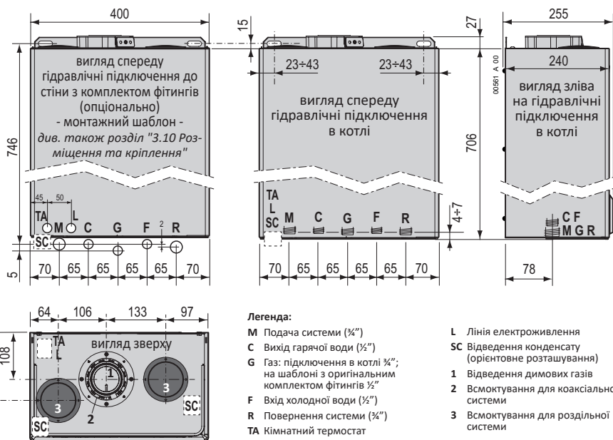
Р.4 - Розміри та підключення
