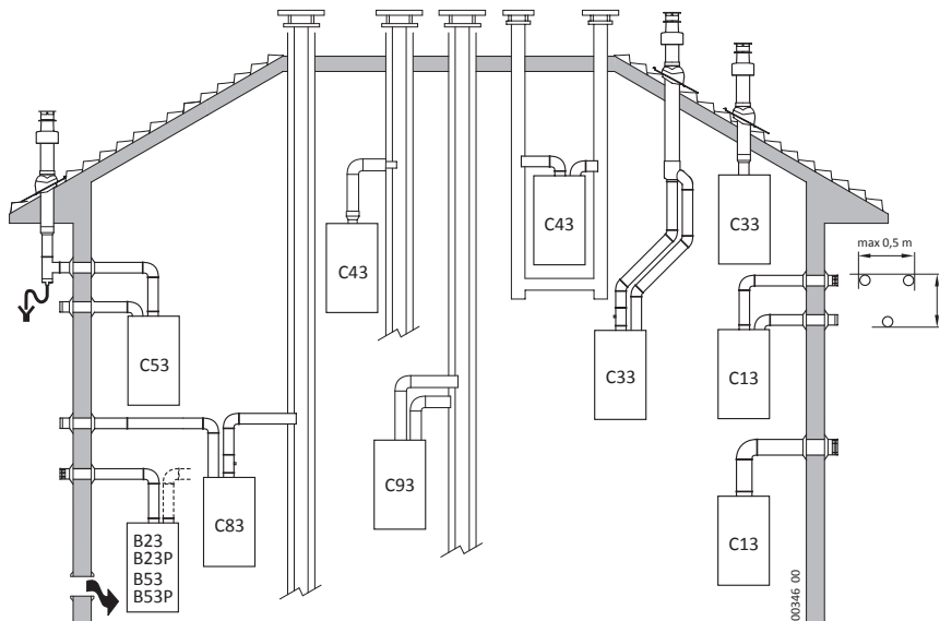
F.14 - Дозволені типи димоходів
