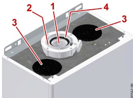
Ф.9 - Випускні/впускні патрубки
