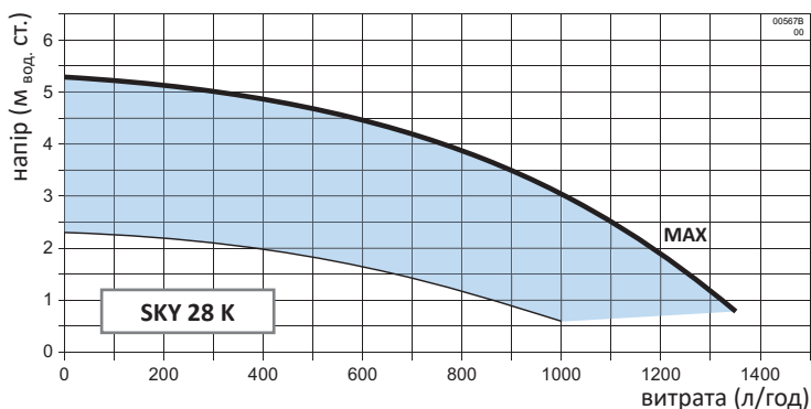
Р.3 - Крива напору SKY 28 K
