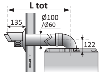
Ф.12 - Приклад горизонтальної коаксіальної системи (C 13 )
