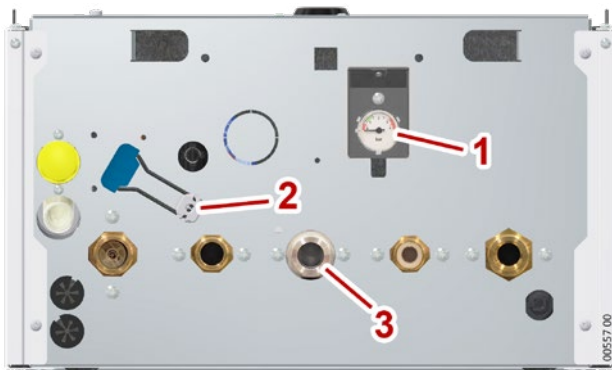
Ф.1 - Елементи керування на нижній стороні
